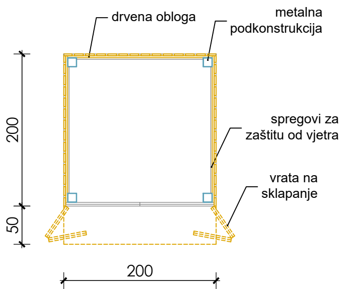
OSNOVA
