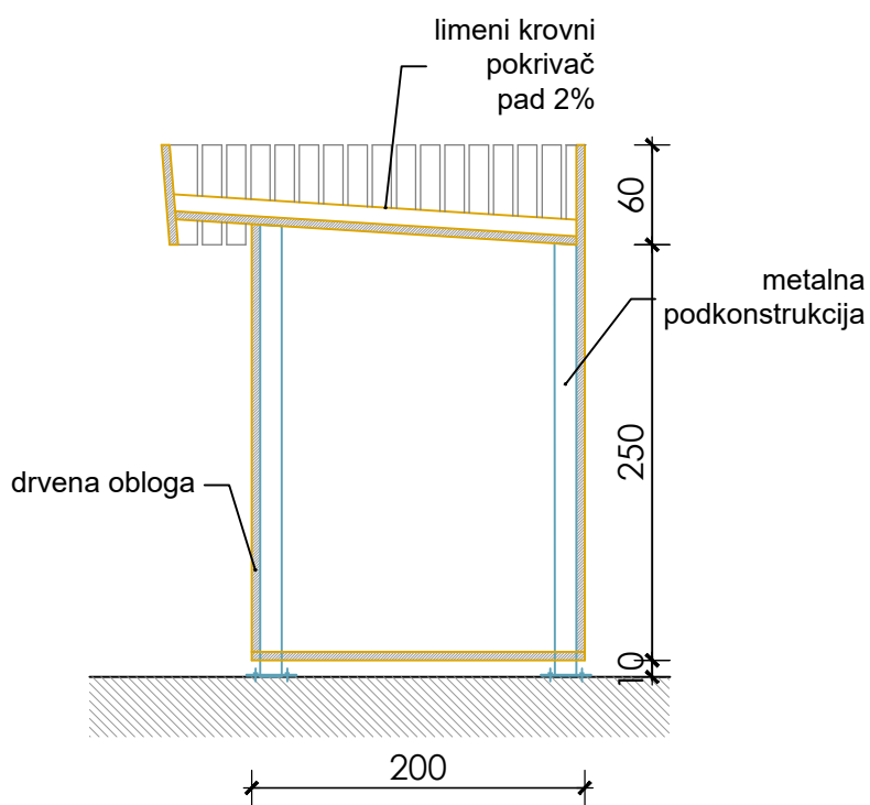
PRESJEK
